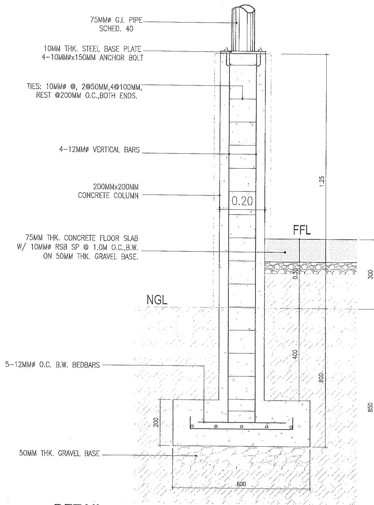
1 F1C1 DETAIL S-3 SCALE 1:10 M.
