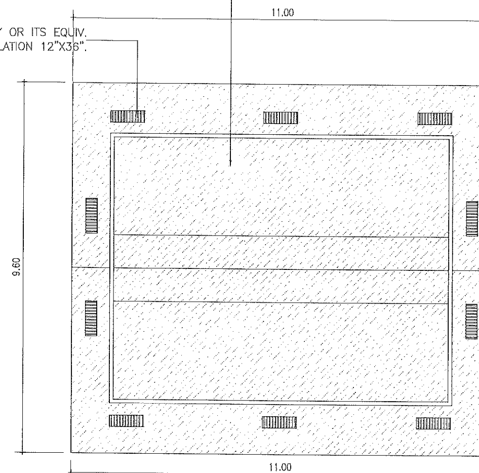
4 CEILING PLAN A-3 SCALE 1:100 M.
