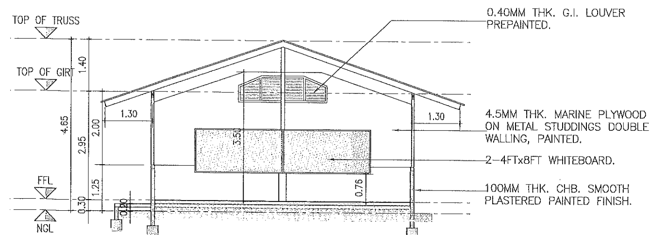
2 CROSS SECTION A-3 SCALE 1:100 M.
