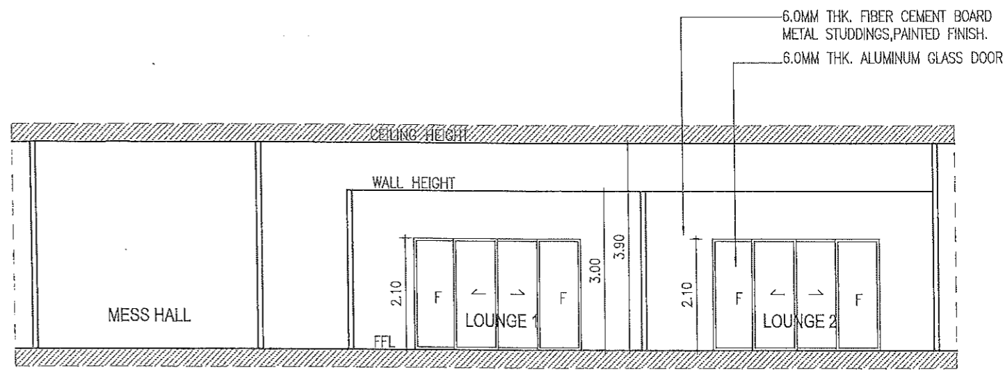
4 SECTION 'B' A-20 SCALE 1:100 M.
