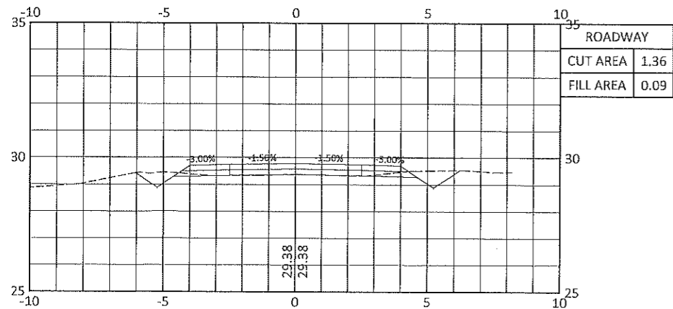
STA. 0+360.00
