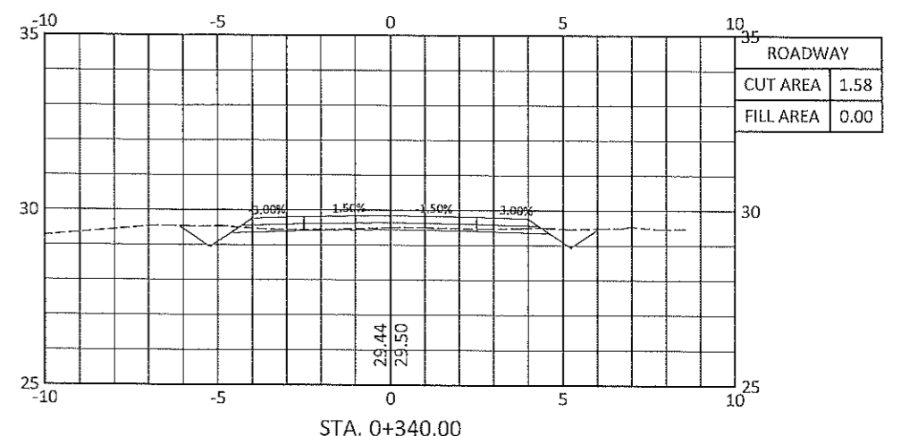
STA. 0+340.00
