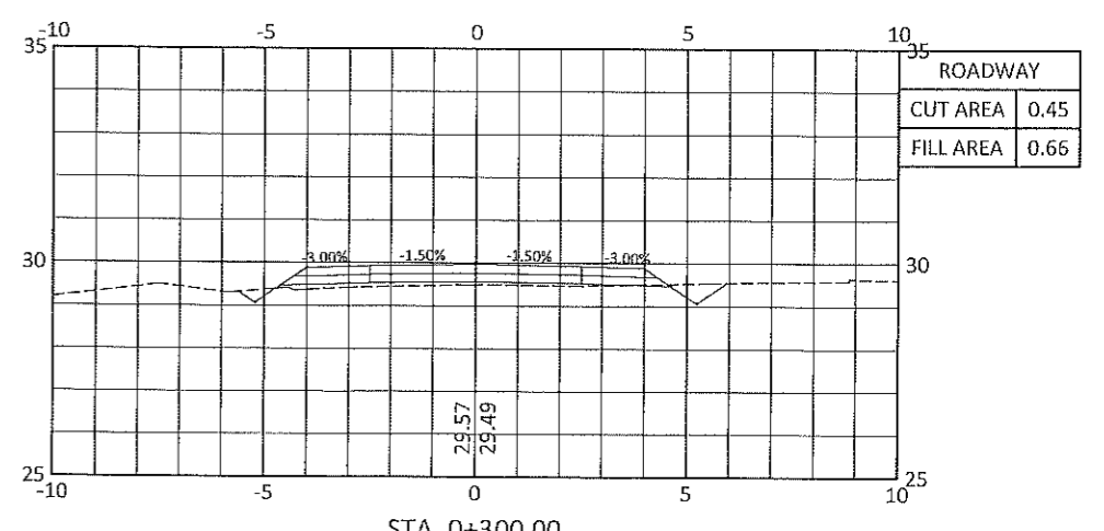
STA. 0+300.00
