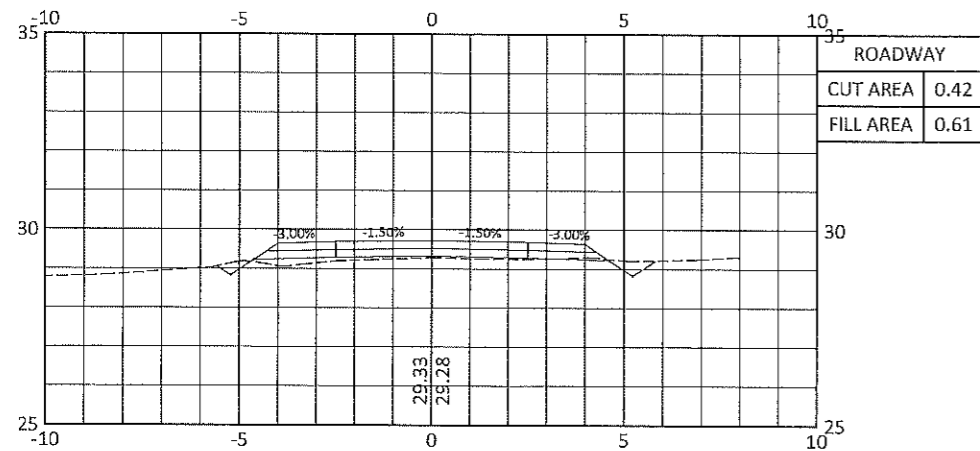
STA. 0+380.00
