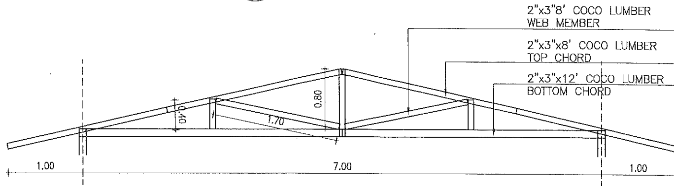
2 TRUSS - 02 A-5 SCALE 1:50 M.
