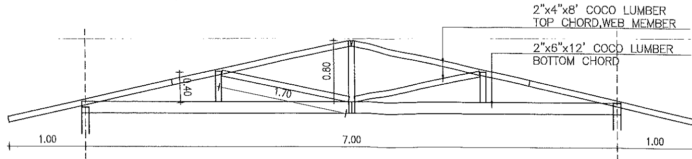
1 TRUSS - 01 A-5 SCALE 1:50 M.
