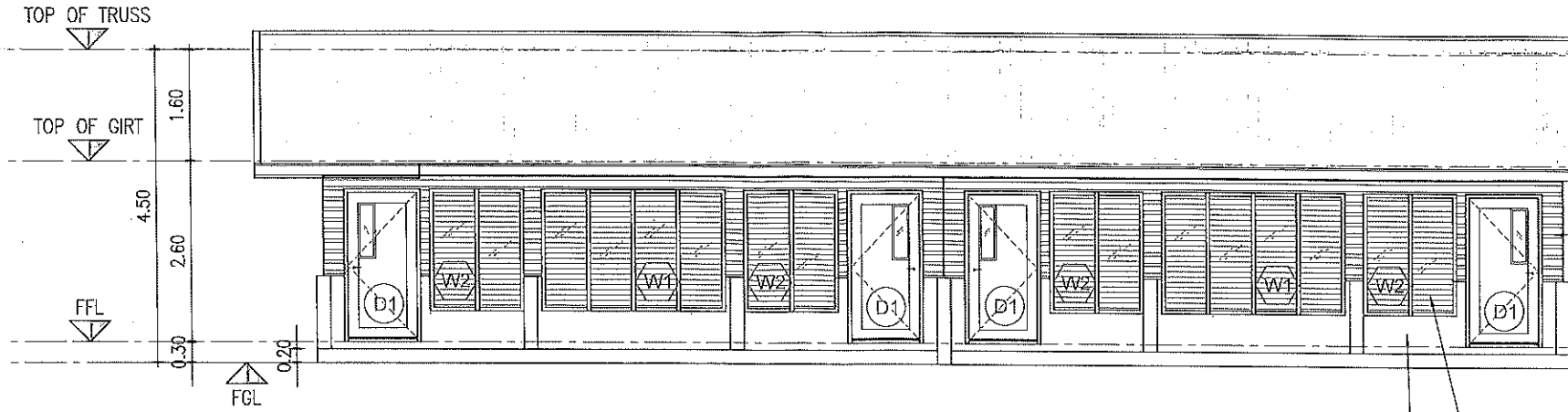
2 FRONT ELEVATION A-2 SCALE 1:100 M.
